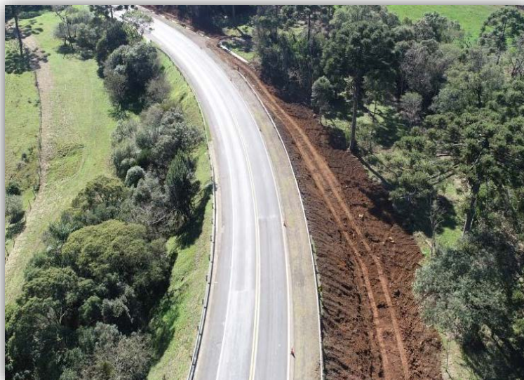
Figura 07 – Execução de Terceiras Faixas – km 156,075 ao 158,245
