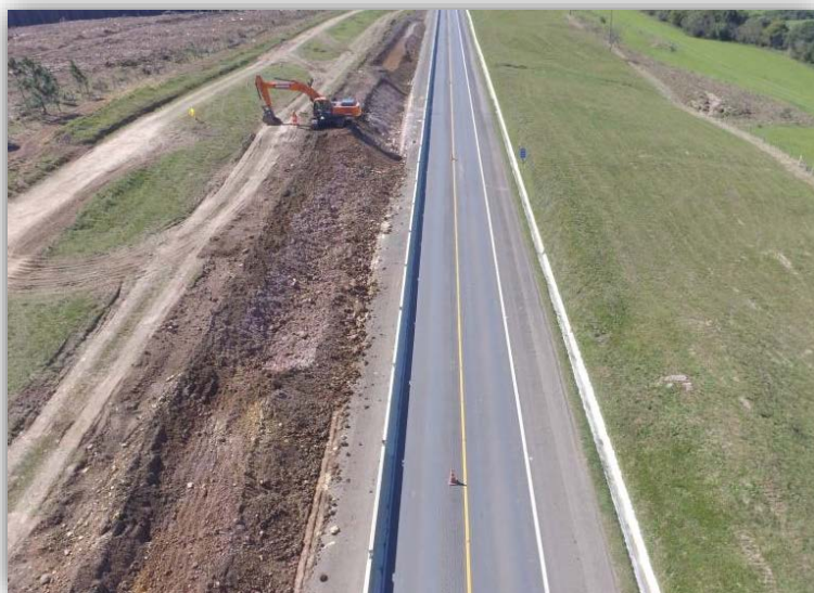
Figura 09 – Execução de Terceiras Faixas – km 212,035 ao 214,185
