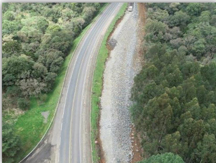
Figura 05 – Execução de Terceiras Faixas – km 124,795 ao 125,810
